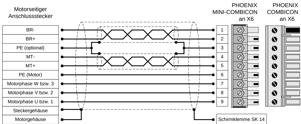
Abbildung 15: Motoranschluss [X6]
