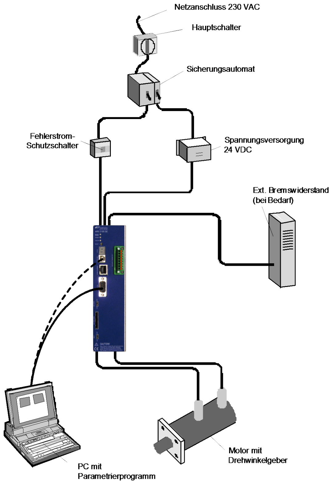
Abbildung 13: Gesamtaufbau ARS 2100 SE (Beispiel mit STO) mit Motor und PC
