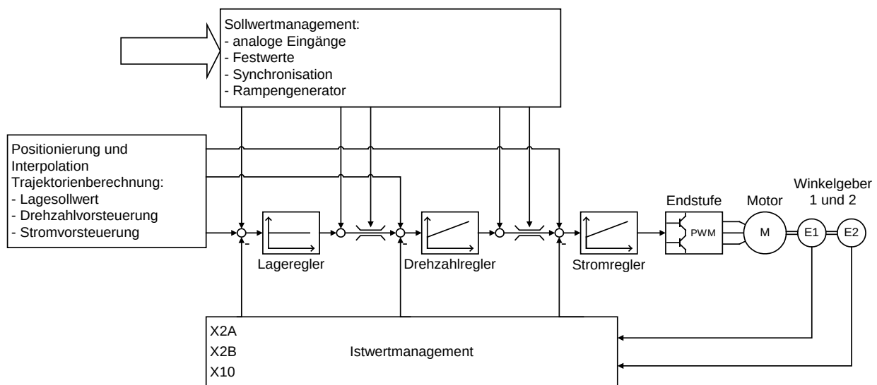
Abbildung 2: Regelstruktur des ARS 2100 SE
