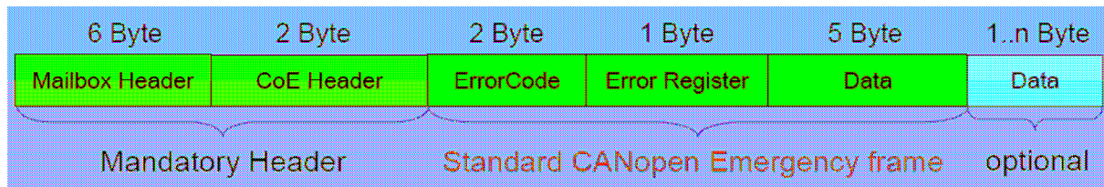
Abbildung 11: Emergency Frame: Telegrammaufbau
