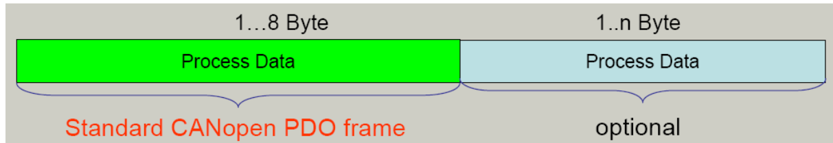
Abbildung 9: PDO Frame: Telegrammaufbau
