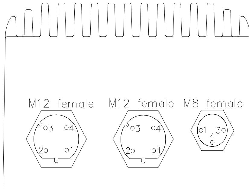
Abbildung 1: Steckerbelegung: EtherCAT
