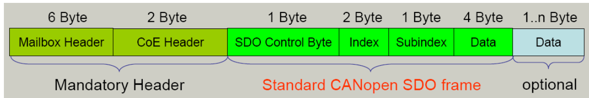
Abbildung 8: SDO Frame: Telegrammaufbau
