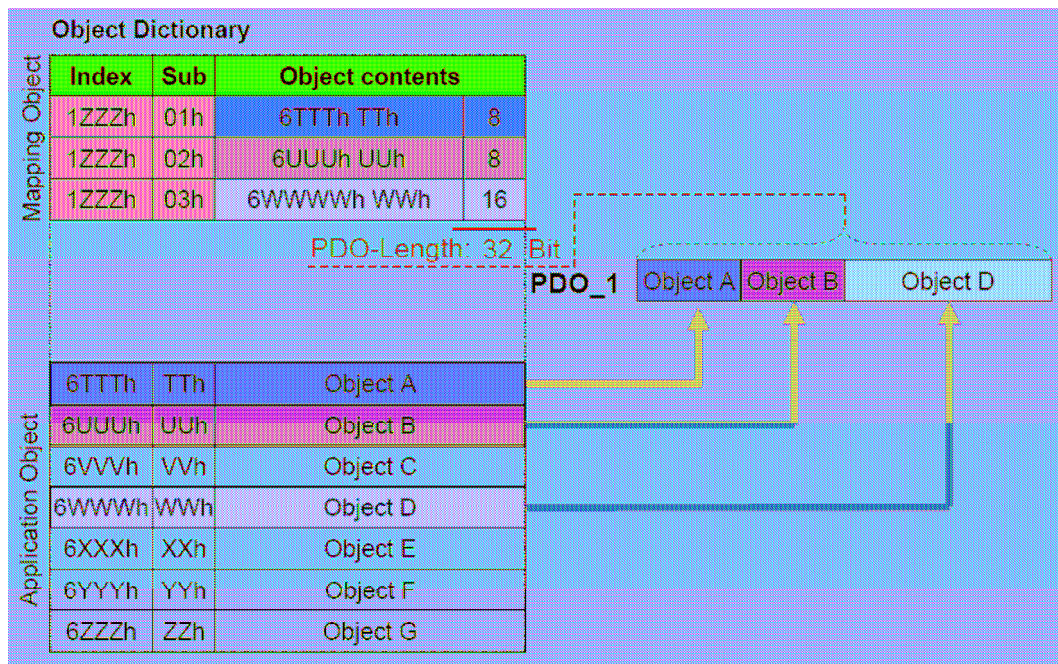
Abbildung 10: PDO-Mapping
