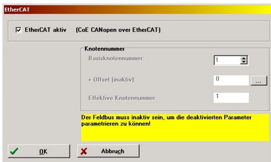
Abbildung 12: Einstellung der EtherCAT-Schnittstelle
