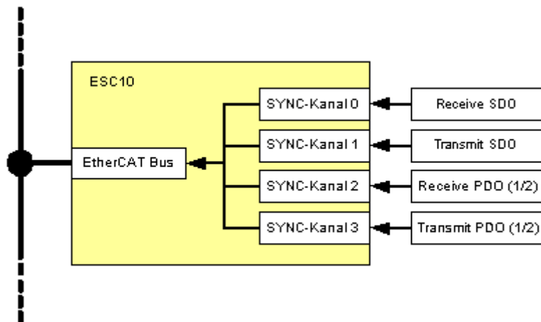
Abbildung 5: Beispielmapping der SDOs und PDOs auf die Sync-Kanäle
