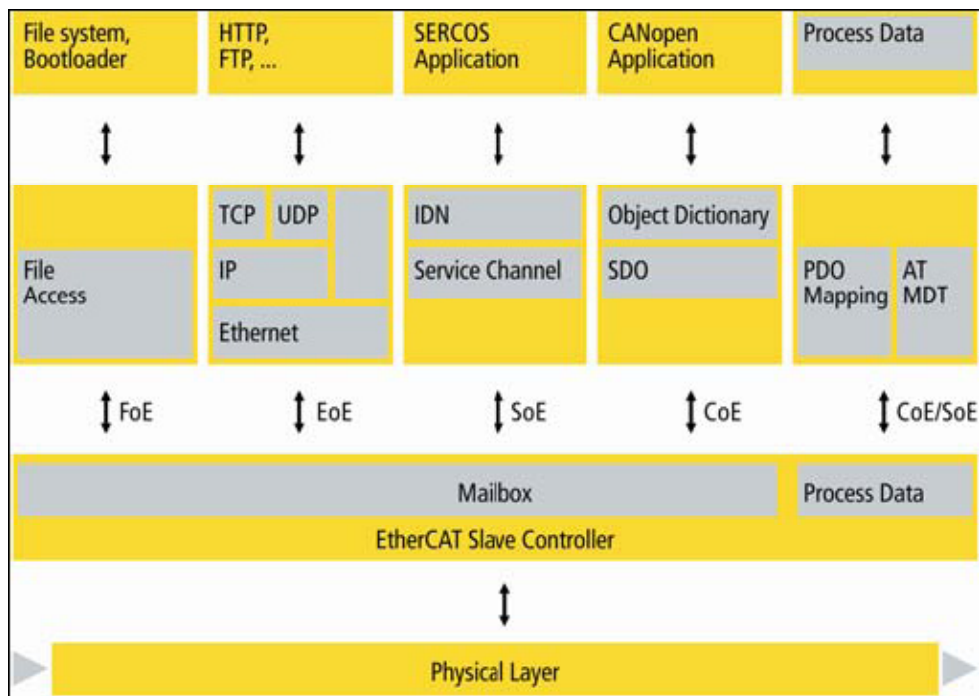
Abbildung 2: Multiprotokollfähiges Feldbussystem EtherCAT
