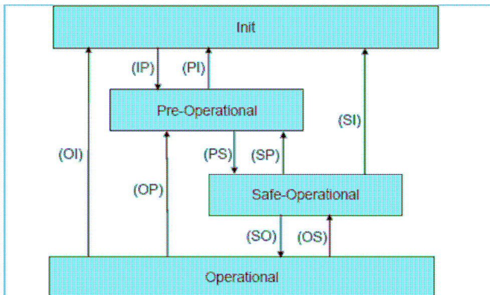
Abbildung 6: EtherCAT Statemachine
